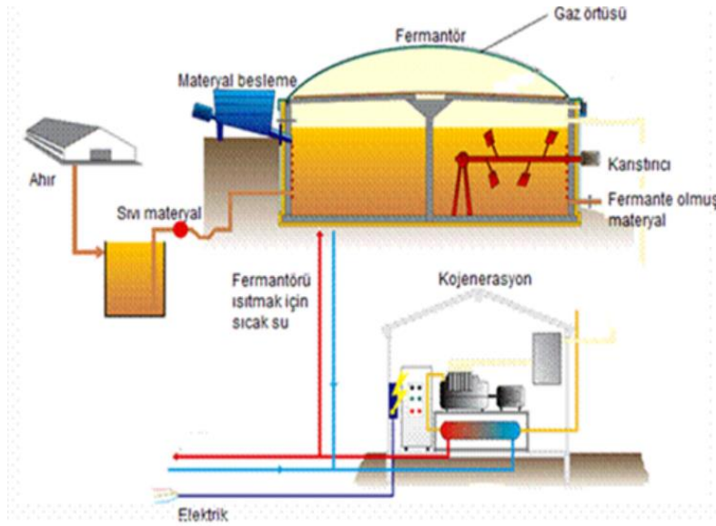
Şekil 5. Biyogaz Elektrik Üretim Tesisi
